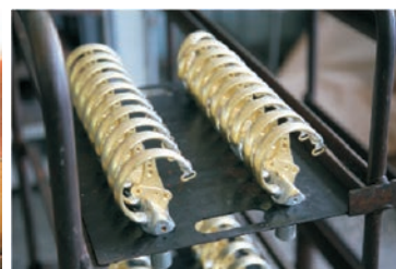
Участок сборки технических манометров
